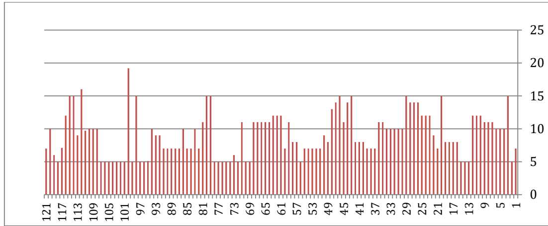
شكل (2) : يوضح عمق النشاط الزلزالي لكل هزة أرضية في منطقة الدراسة للفترة (1984-2024)
