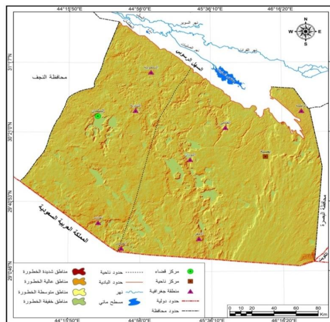
خريطة (6) التوزيع المكاني للمخاطر المورفومناخية في بادية محافظة المثنى
