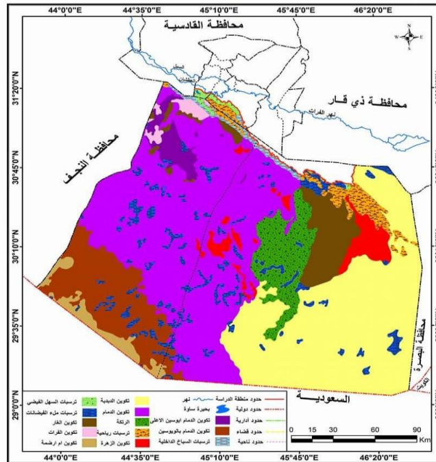
الخريطة (2) التكوينات الجيولوجية في بادية محافظة المثنى
