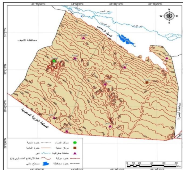
خريطة (3) خطوط الارتفاع المتساوي /م في بادية المثنى
