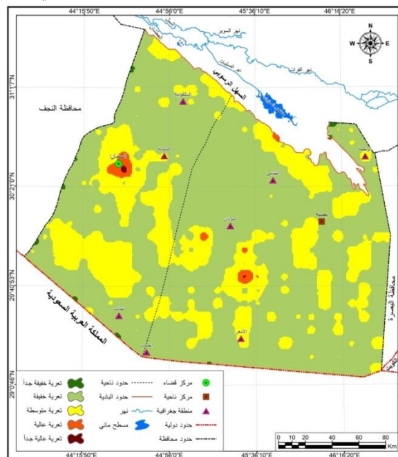
الخريطة (5) انطقه التعرية المائية وفق تصنيف (Bergsma) في بادية المثنى
