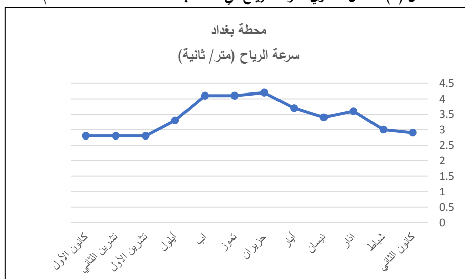
الشكل (٣) المعدل السنوي لسرعة الرياح في محطة بغداد للمدة ٢٠١٤ - ٢٠٢٤م
