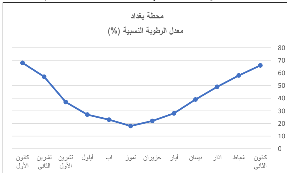
المعدل السنوي للرطوبة النسبية في محطة بغداد للمدة ٢٠١٤ - ٢٠٢٤م
