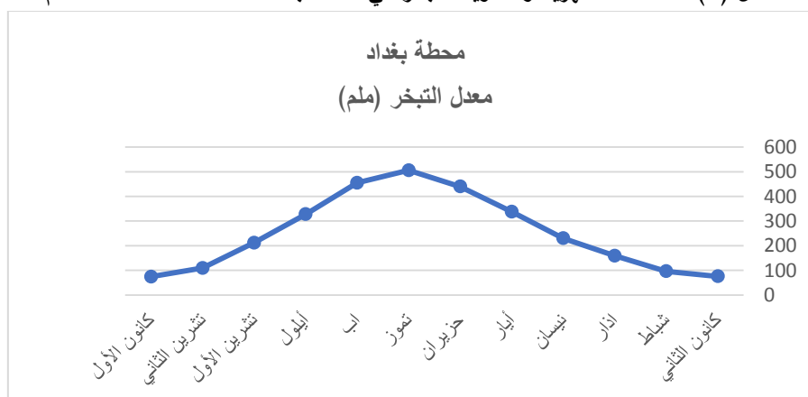
الشكل (٦) المعدلات الشهرية والسنوية للتبخر في محطة بغداد للمدة ٢٠١٤ - ٢٠٢٤ م
