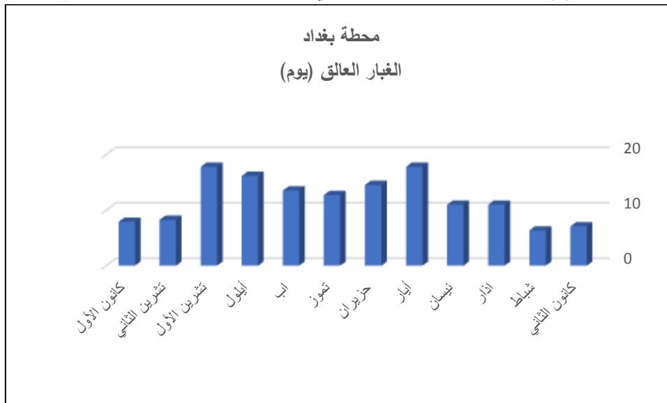
الشكل (٨) المعدلات الشهرية للغبار العالق في محطة بغداد للمدة ٢٠١٤ - ٢٠٢٤ م
